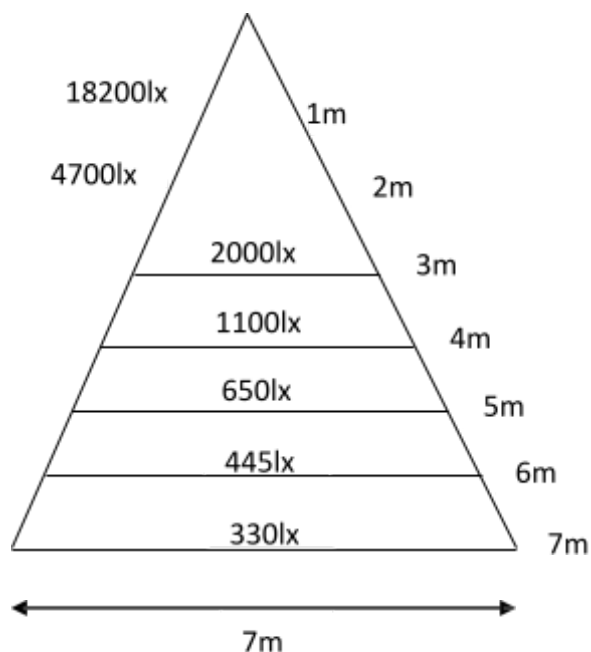
Distribución de Iluminancia
